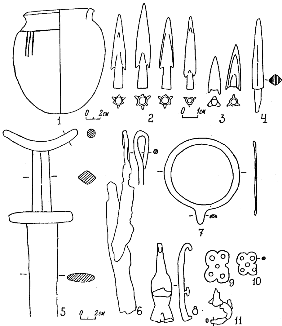
Рис. 9. Тамбовский могильник. Курган 2. Вещи из погребения 6: 1-сосуд, 2-4 - наконечники стрел, 5- меч, 6- ножи, 7- зеркало, 8- колчанный крючок, 9-10 - портупейные обоймы, 11 - пряжка (1- глина, 2, 4-6, 8-11 - железо, 3, 7- бронза).
